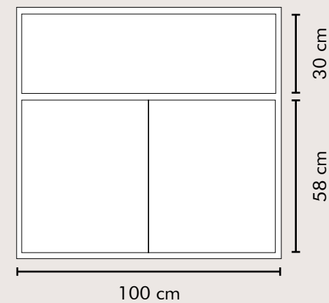
VUE DE DOS tablette + placards avec serrure
