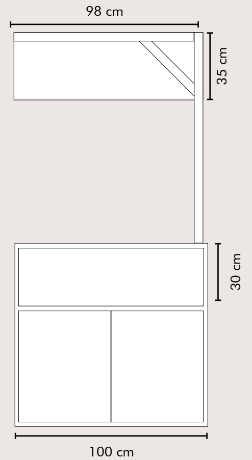
VUE DE DOS tablette + placards avec serrure
